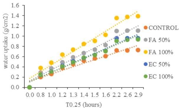
Gambar 6. Hasil uji serapan \text{Na}_2\text{SO}_4 kapiler beton
