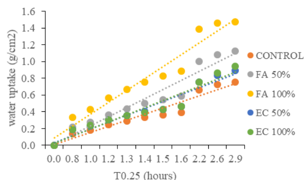
Gambar 6. Hasil uji serapan NaCL kapiler beton
